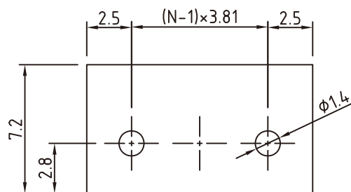
P.C.B. LAYOUT
