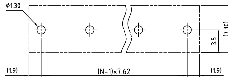
P.C.B. LAYOUT
