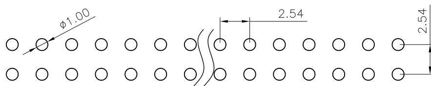
P.C.B LAYOUT
