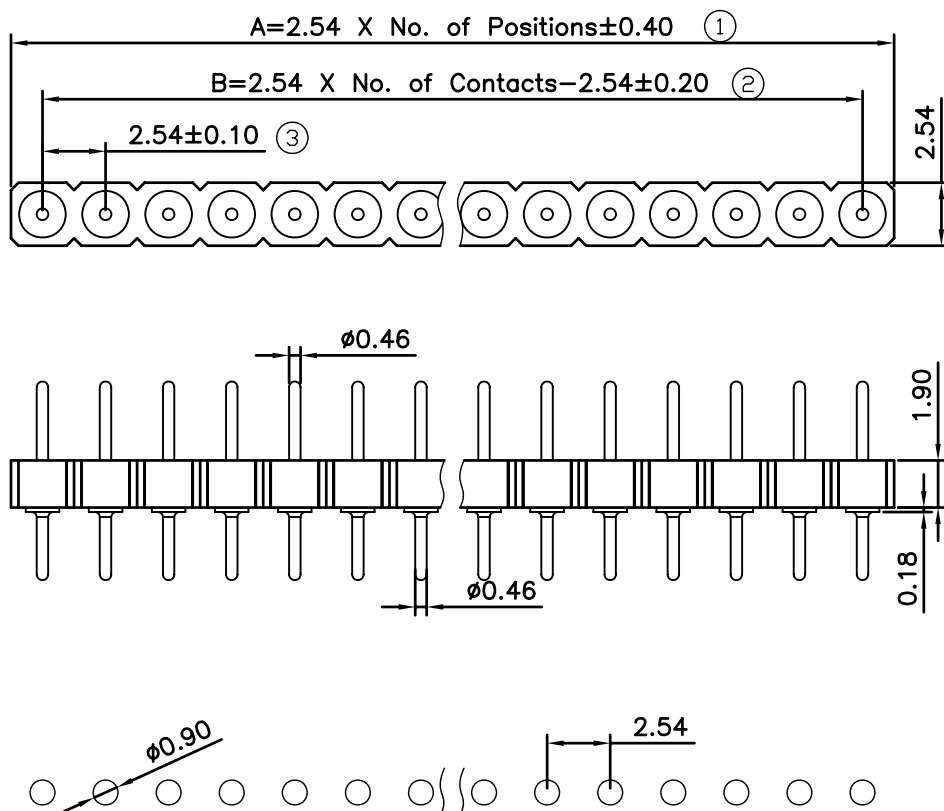
P.C.B LAYOUT
