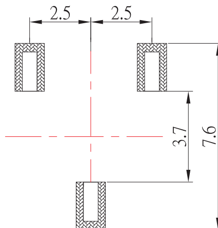
P.C.B LAND PATTERN
