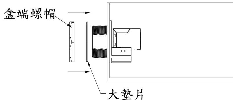
防水盒端
