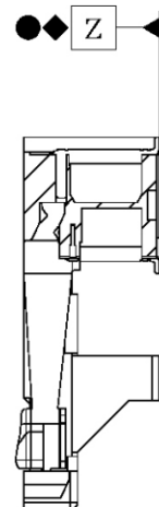
A-A (2 : 1)
