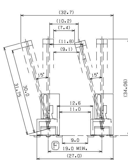
推奨 SOCKET レイアウト寸法
