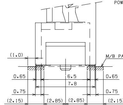
コンタクト接地長
