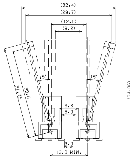
推奨 SOCKET レイアウト寸法
