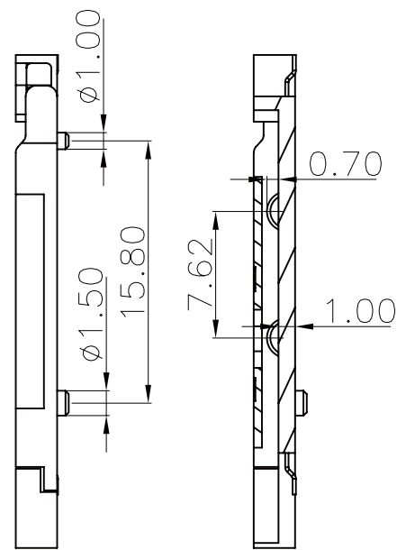
SECTION:X-X
