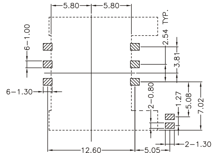
P.C.B LAYOUT TOP VIEW \pm 0.05
