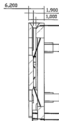
剖面 B-B 比例 1:1
