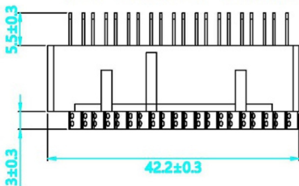
端子 銅 鍍鎳 T=0.3MM
