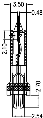
SECT A-A
