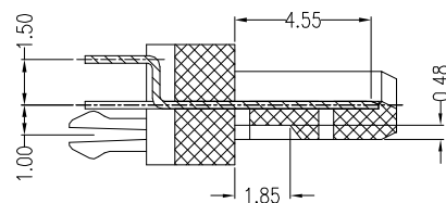
SECT A-A
