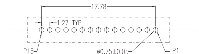
P.C.B LAYOUT(T=1.60mm) COMPONENT SIDE
