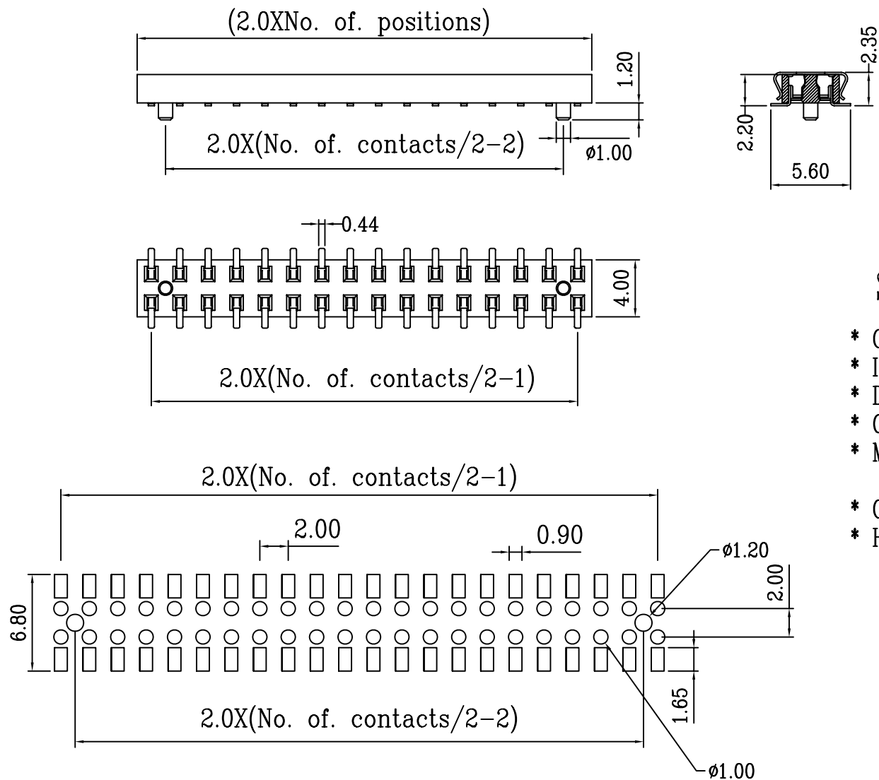
P.C.B. layout
