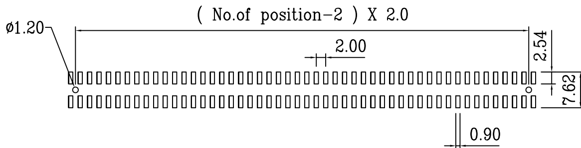
P.C.B.layout
