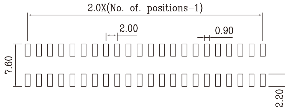
P.C.B. layout
