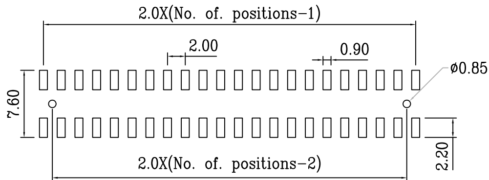
P.C.B. layout
