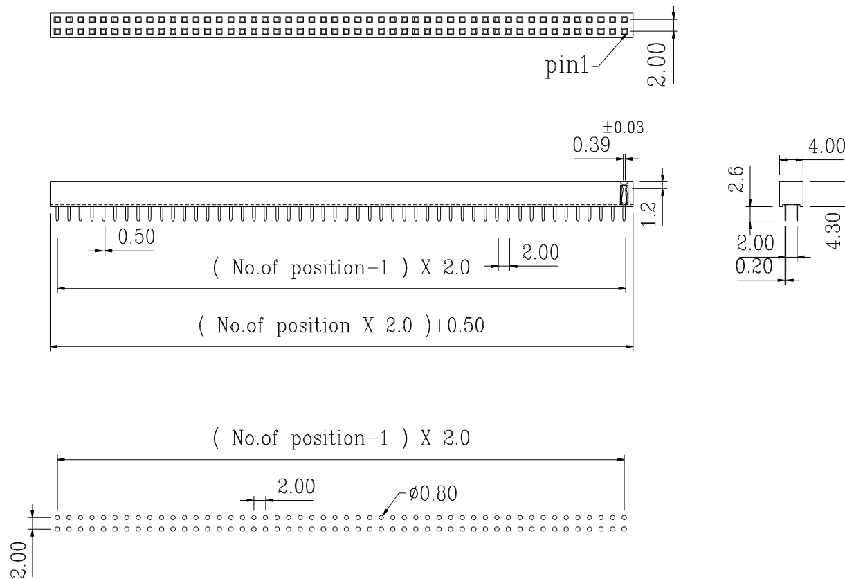
P.C.B.layout
