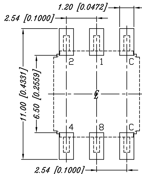
P.C.B. LAYOUT
