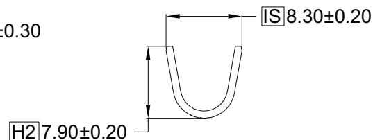
剖面 B-B
