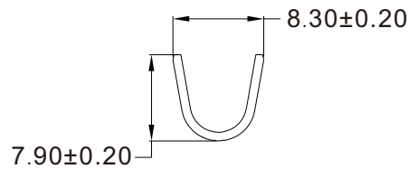
剖面 B-B
