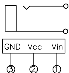
电路图
