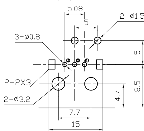
印制板开孔图
