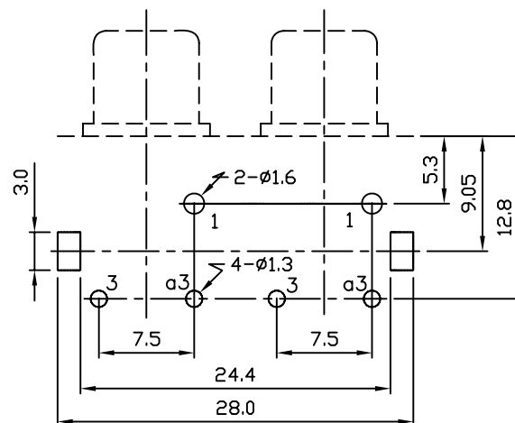
P.C.B LAYOUT(±0.1) BOTTOM VIEW
