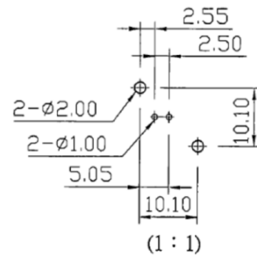
(1 : 1) P.C.B. LAYOUT (印刷电路板配置)
