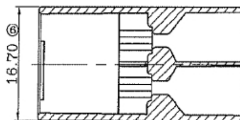
SEC A-A
