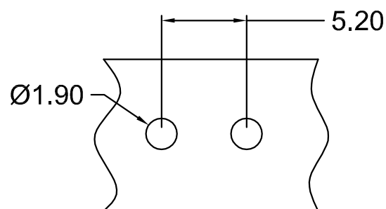
PCB孔尺寸
