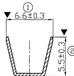
SEC. A-A
