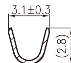
SEC.B-B
