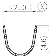
SEC A-A
