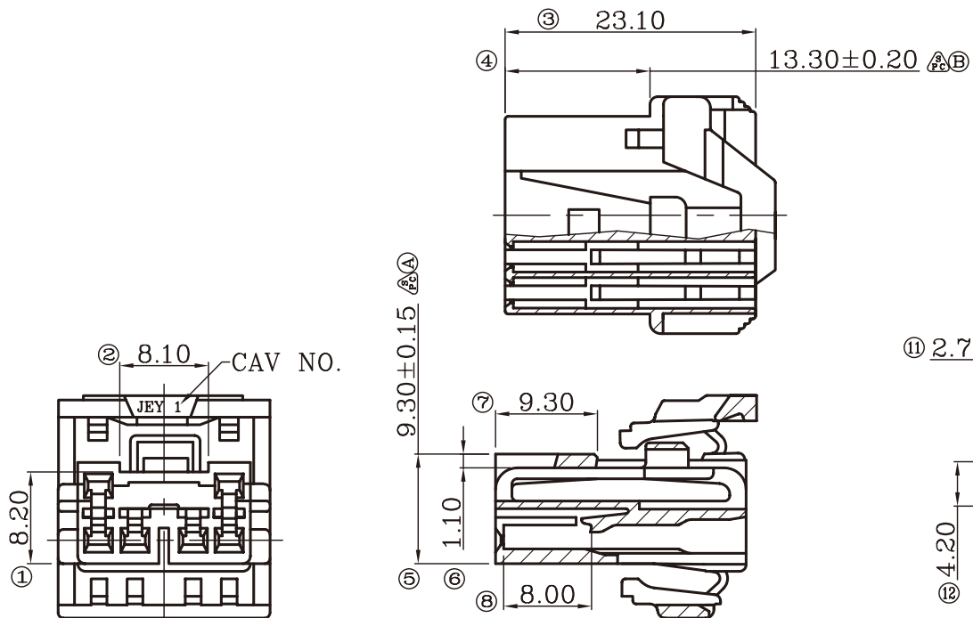
SEC A-A
