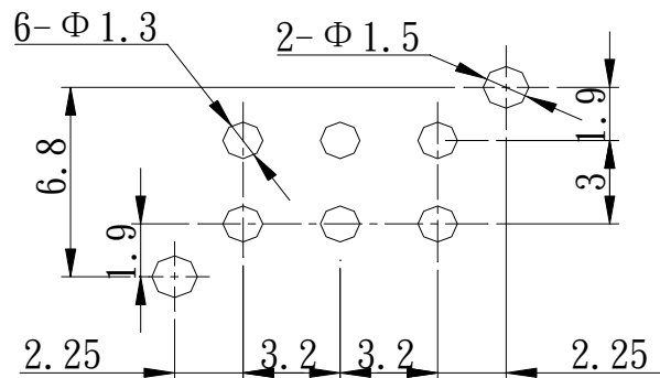
P.C.B HOLE DETAL
