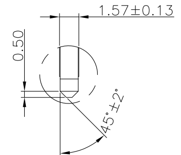
DETAIL:A-A SCALE :2:1
