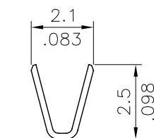
SEC.: A-A
