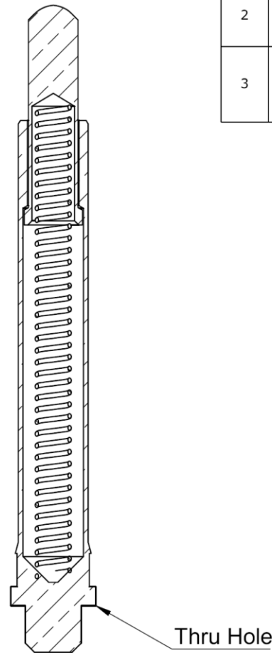
SECTION B-B SCALE 10 : 1
