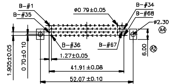
P.C.Board Layout
