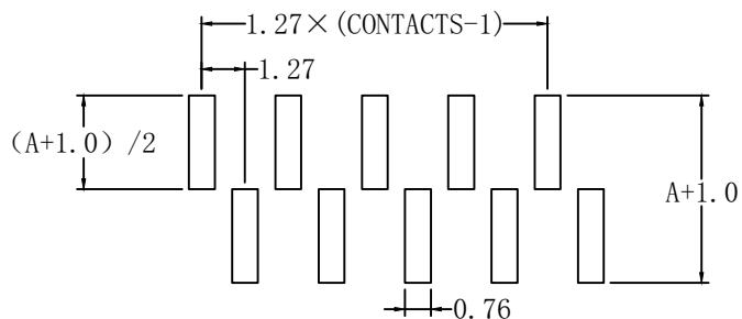
P. C. B. LAYOUT
