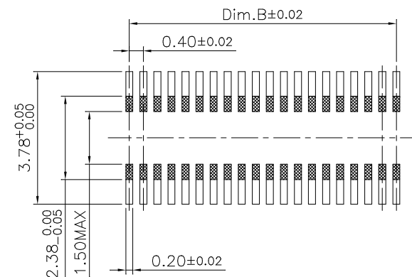
P.C.B Layout
