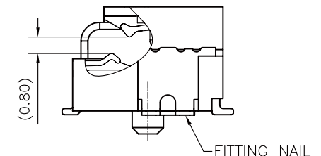
SECTION A-A Scale 4:1
