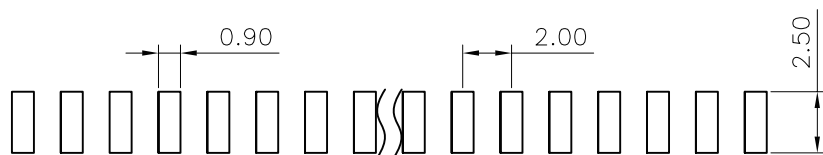
P.C.B LAYOUT
