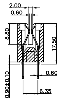
SEC A-A
