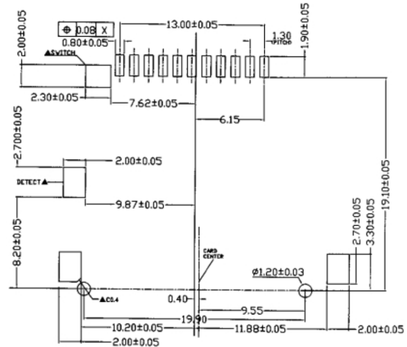
P.C.B layout
