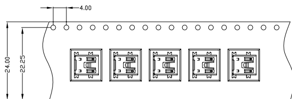
① 载带
