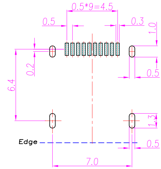
Recommend P.C.B Layout.
