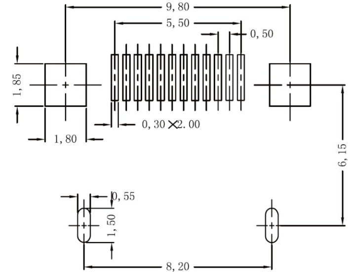
P.C.B. Layout
