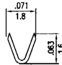
A-A SECTION
