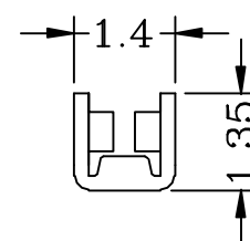
Section D-D
