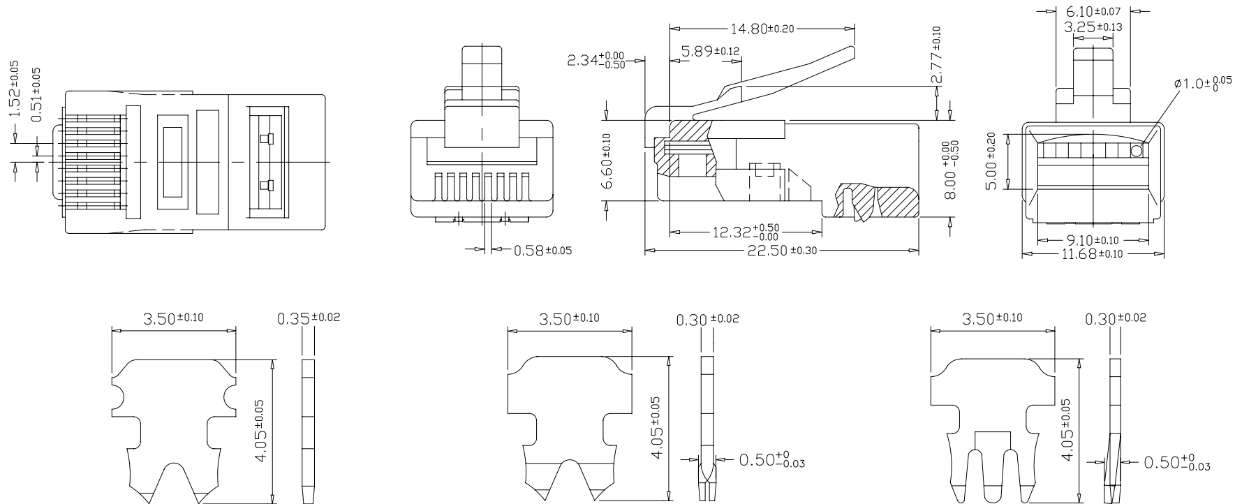
2 PRONGS FOR STRANDED WIRE 多芯線用二叉型金片 (MP-R-0808B)
