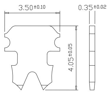
“ ” : 2PRONGSFOR STRANDED WIRE 多芯線用二叉型金片
